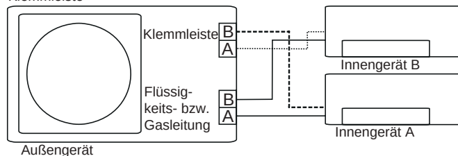
Klemmleiste
