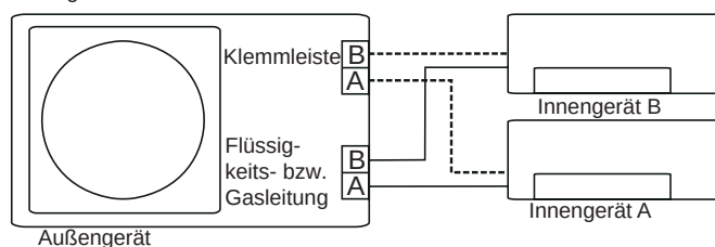
Klemmleiste
