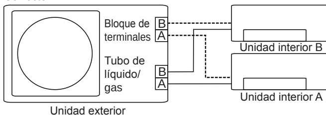
Cableado incorrecto
