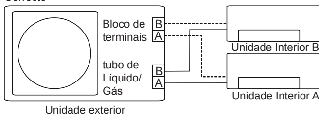
Cablagem incorreta
