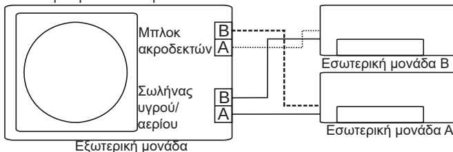
Λανθασμένη καλωδίωση
