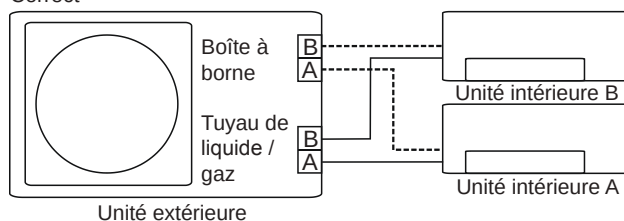
Câblage incorrect
