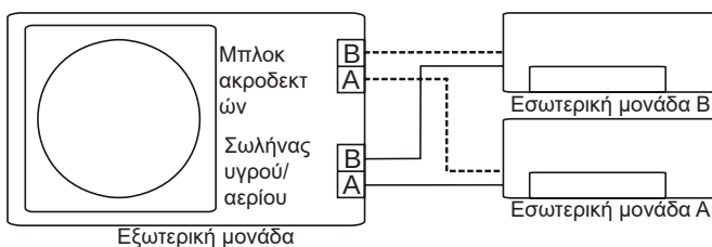
Λανθασμένη καλωδίωση
