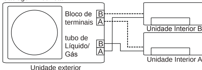
Cablagem incorreta
