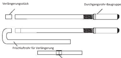
Schnittstelle von zwei Rohrverbindungen
