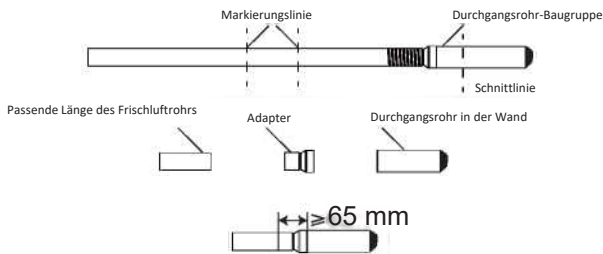
Frischluftrohr, Adapter und Durchgangsrohr anschließen
