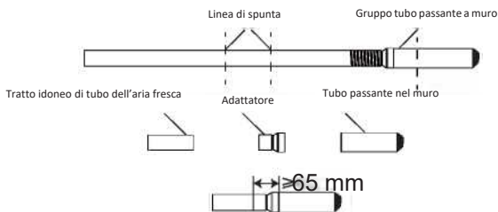
Collegare il tubo dell'aria fresca, gli adattatori e il tubo passante nel muro
