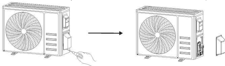
Retirer le couvercle de la valve tuyaux de raccordement
