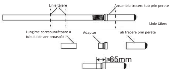
Conectați tubul de aer proaspăt, adaptoarele și tubul de trecere prin perete
